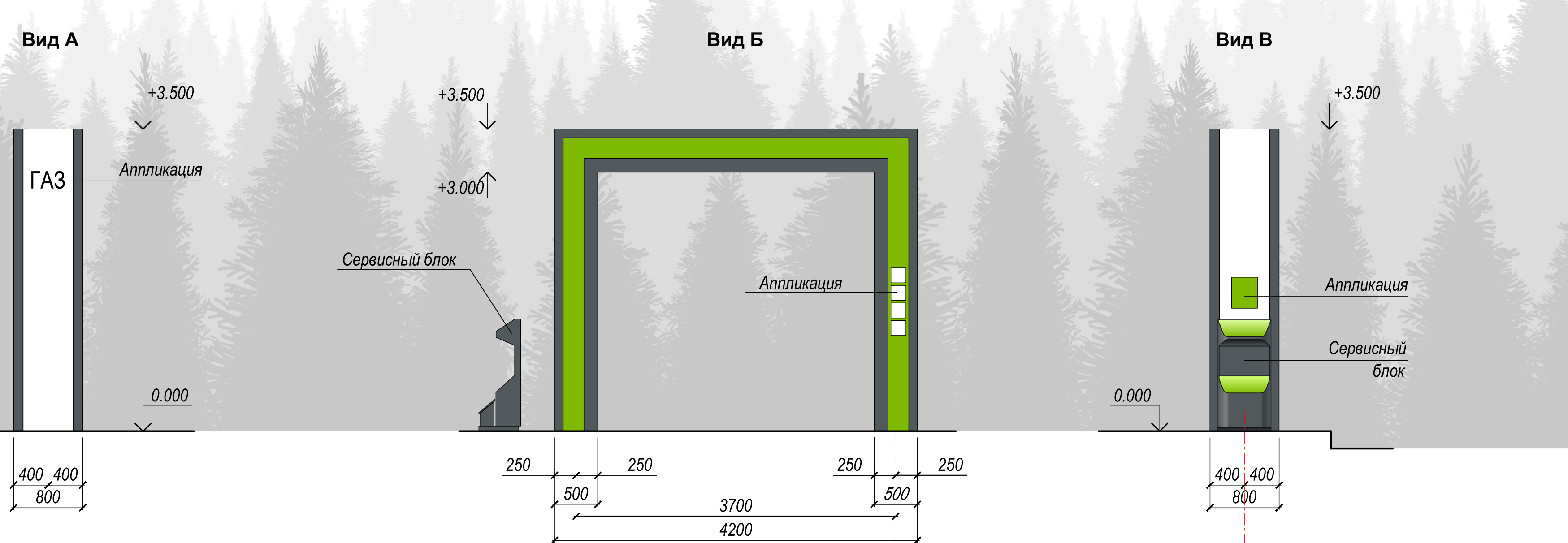
ЗДАНИЕ АЗС
